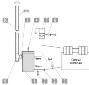
б) открытая система с самоточной циркуляцией
