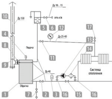
а) открытая система с принудительной циркуляцией
