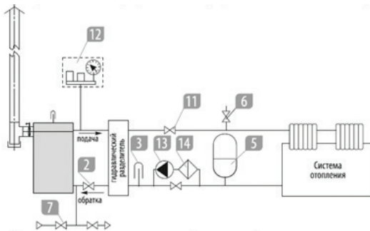
в) закрытая система с принудительной циркуляцией
